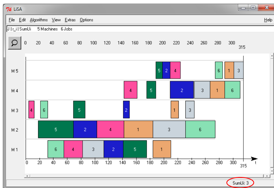
Rys. 2.5. Rezultat harmonogramowania z użyciem algorytmu Tabu Search – wykres Gantta
