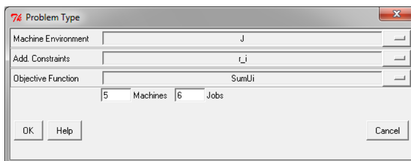
Rys. 2.2. Okno definiowania typu problemu harmonogramowania
